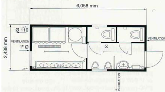
Floor plan Type SA 20':
